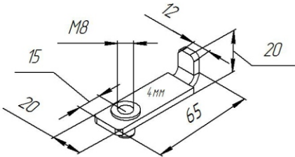
Закладной кронштейн М8 65х20 (поз.5)
