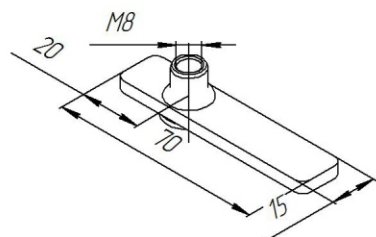
Кронштейн закладной с заклепкой M8 (поз.6)
