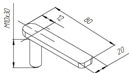
Закладной кронштейн M10 80x20 (поз.7)
