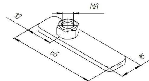
Закладной кронштейн (z-47 M8)(поз.8)
