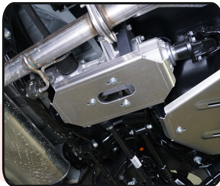
Защита заднего редуктора (алюминий) 4мм арт. ZKTCC00620.
