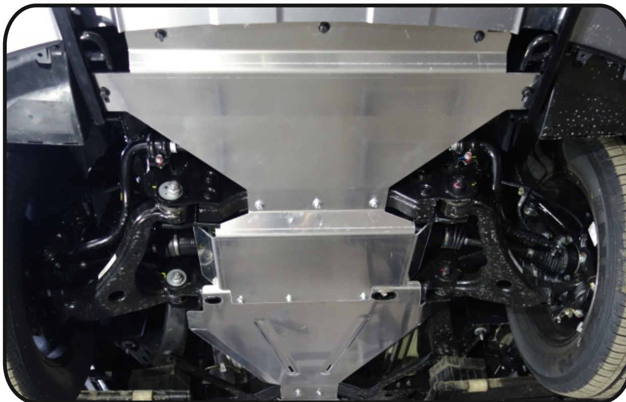
Защита радиатора (алюминий) 4 мм арт.ZKTCC00300.
