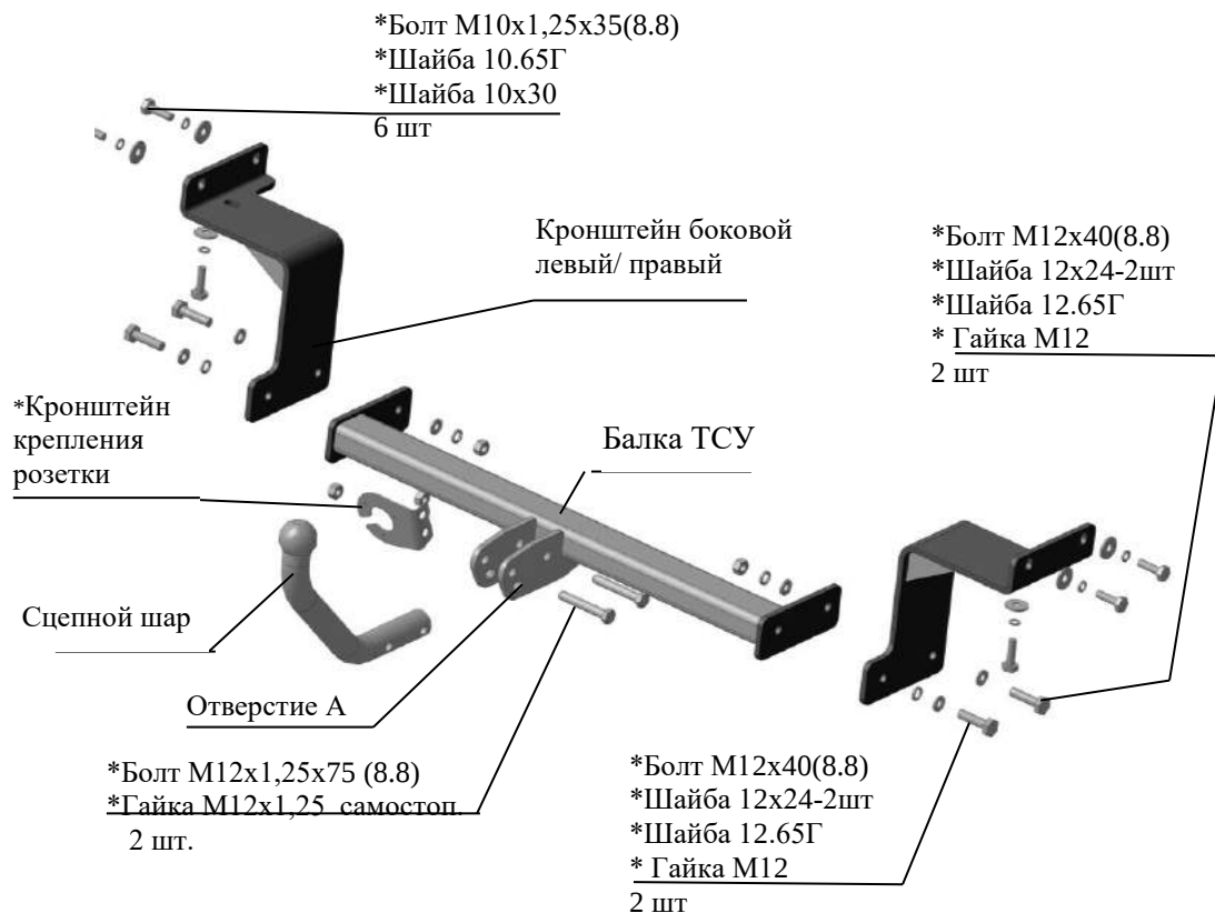
Рис.1 Тягово-сцепное устройство 7354.
